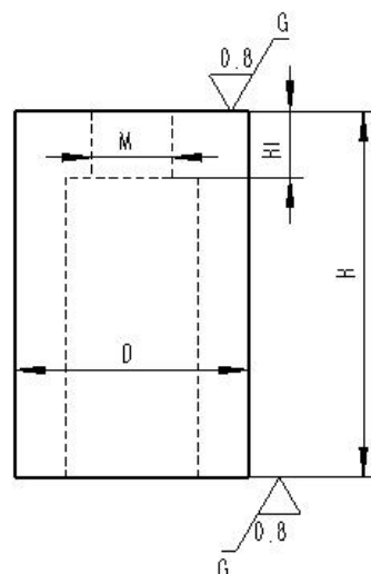
选型示意图
